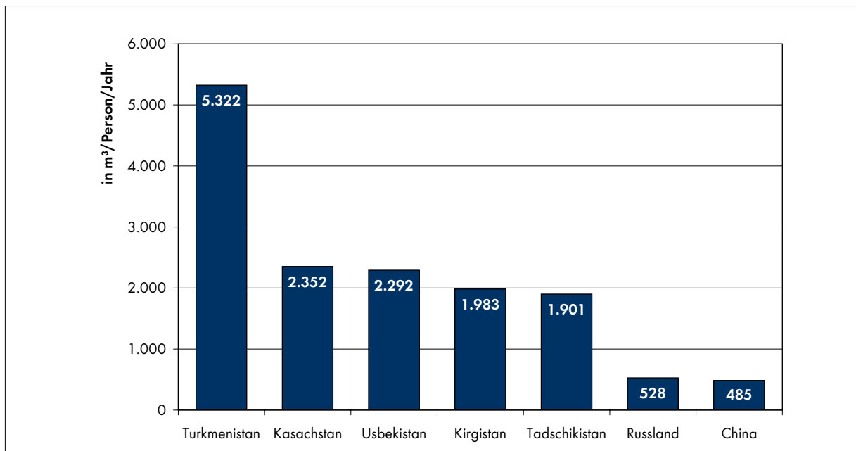
Wasserentnahme absolut 1998–2002 ((in m 3 /Person/Jahr)
